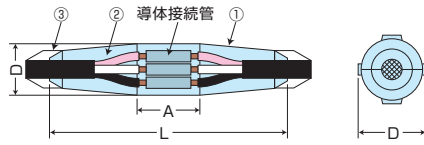
①ケース ②ウレタン系レジソ ③シーリングテープ
