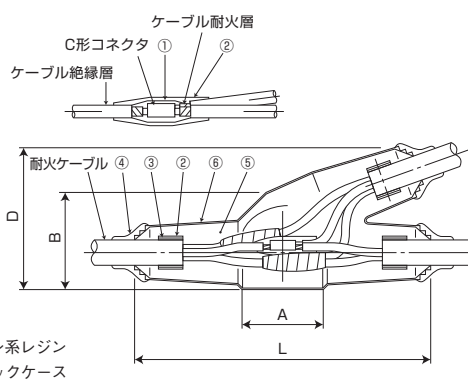
耐火用セルパック Y分岐接続用キット
